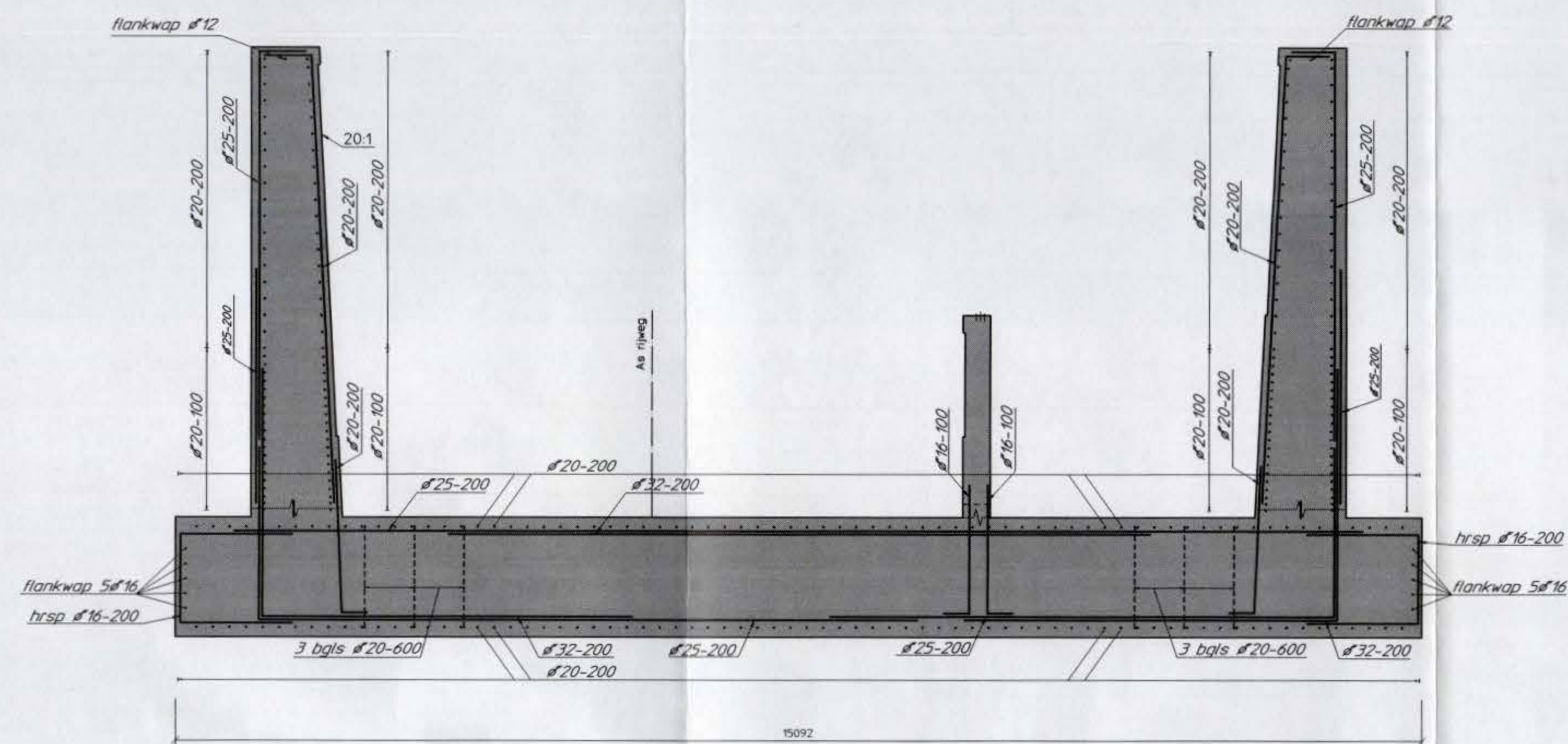
Doorsnede E-E
