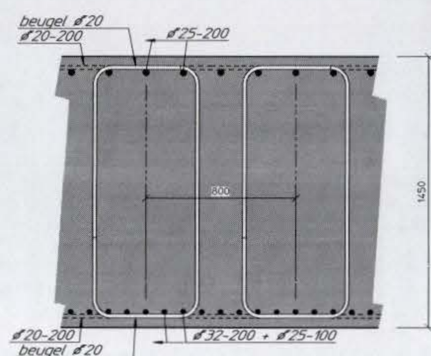
Doorsnede G-G
