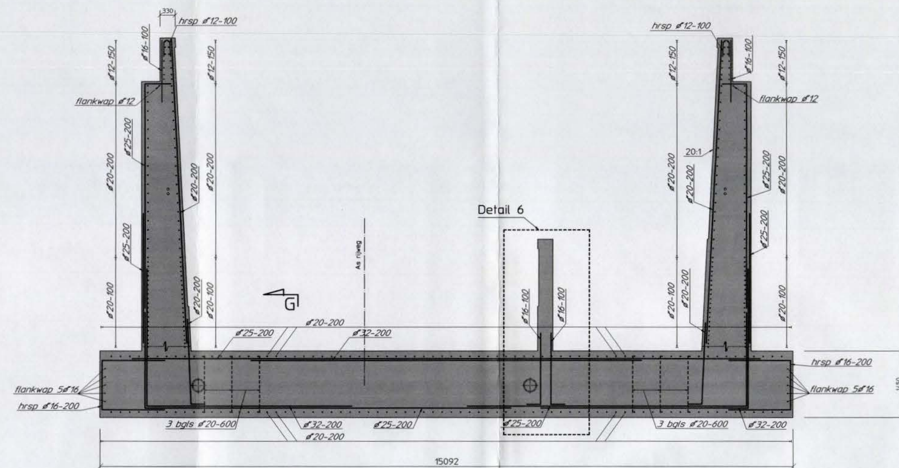
Doorsnede F-F
